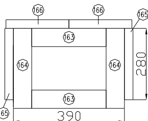
Šamotová vyzdívka
